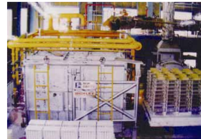
ガイシ用シャトルキルン
